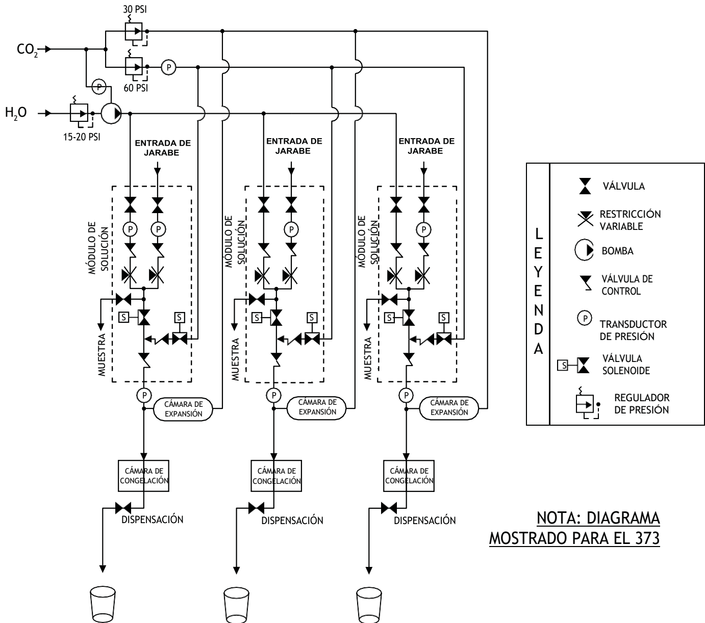
Figura 11.4 Diagrama de flujo de los dispensadores estándar 372 y 373
