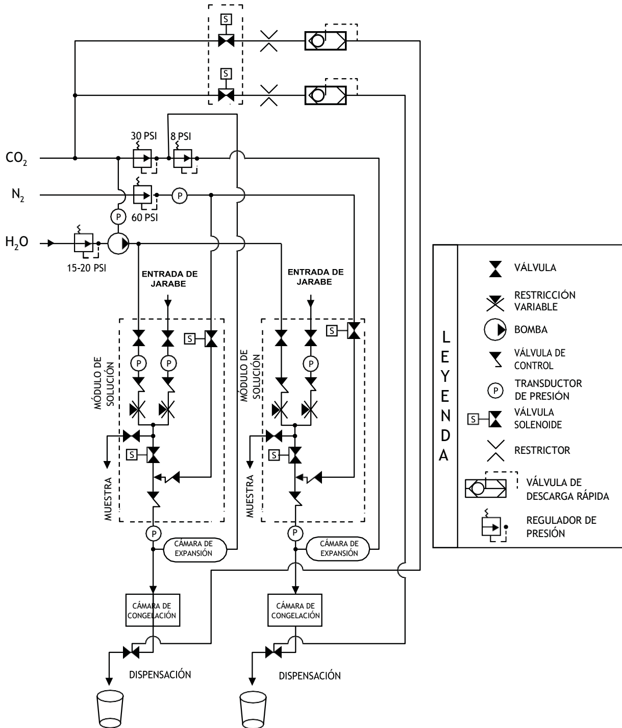
Figura 11.5 Diagrama de flujo del dispensador de nitro 372
