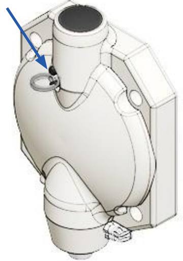
Figura 5.3 Ubicación de la válvula de alivio en varios tipos de placas frontales
