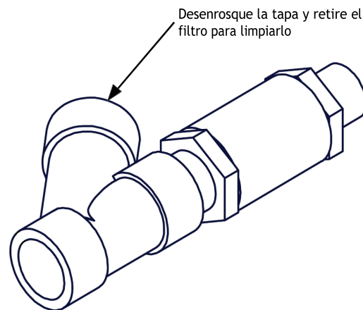
Figura 9.2 Válvula antirretorno
