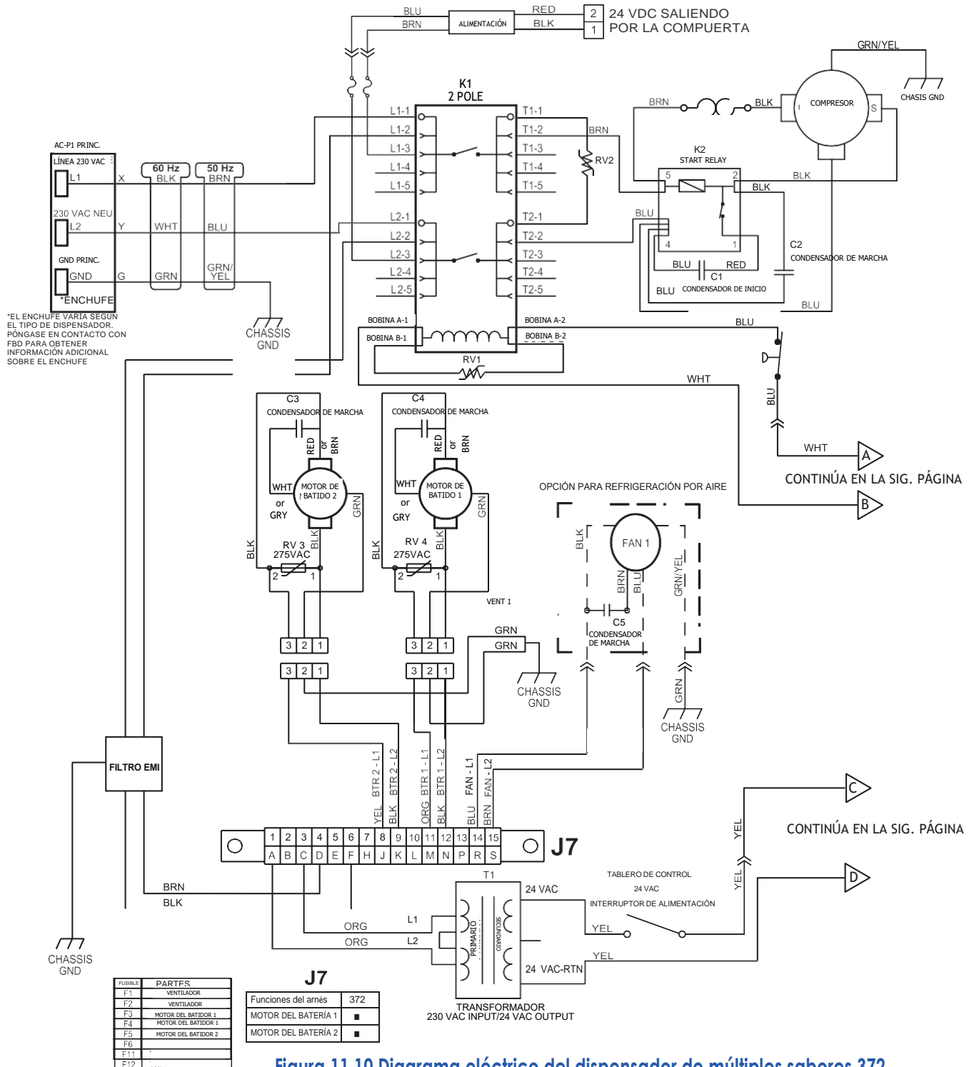
Figura 11.10 Diagrama eléctrico del dispensador de múltiples sabores 372
