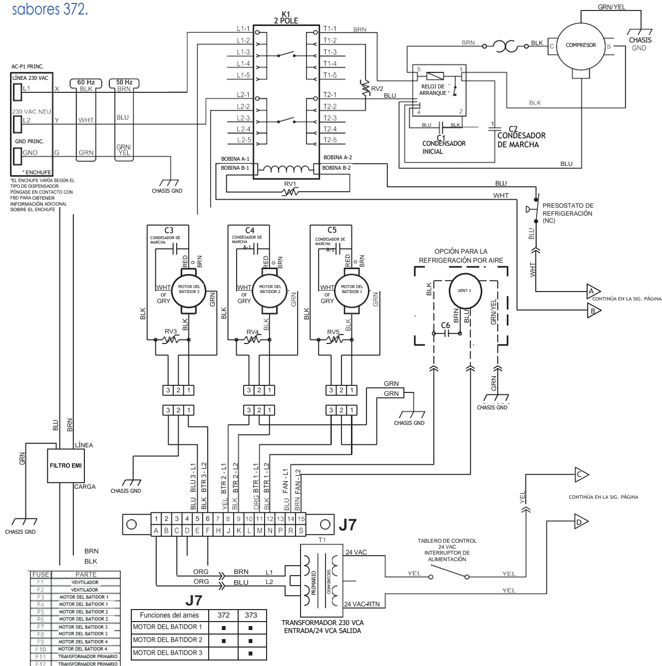
Figura 11.7 Diagrama eléctrico del dispensador estándar 372 1 DE 3
