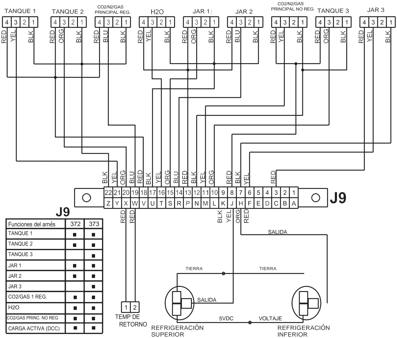
Figura 11.9 Diagrama eléctrico del dispensador estándar 372
