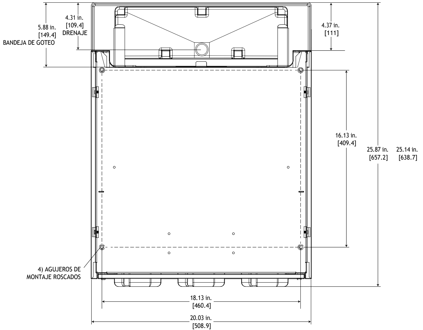
Figura 11.2 Diagrama de montaje del dispensador 373
