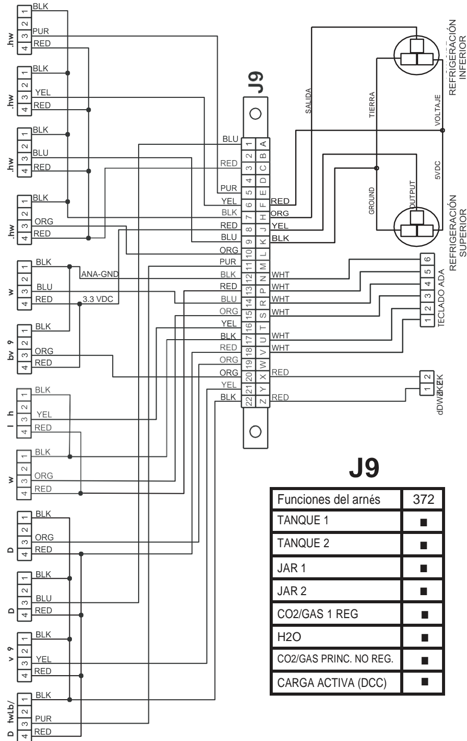
Figura 11.12 Diagrama eléctrico del dispensador de múltiples sabores 372 3 DE 3
