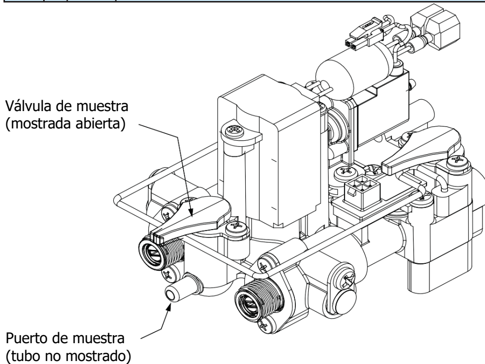
Figura 5.1 Válvula de muestra en el módulo de solución
