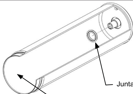
Parte delantera del barril (placa frontal y barra batidora retiradas)
