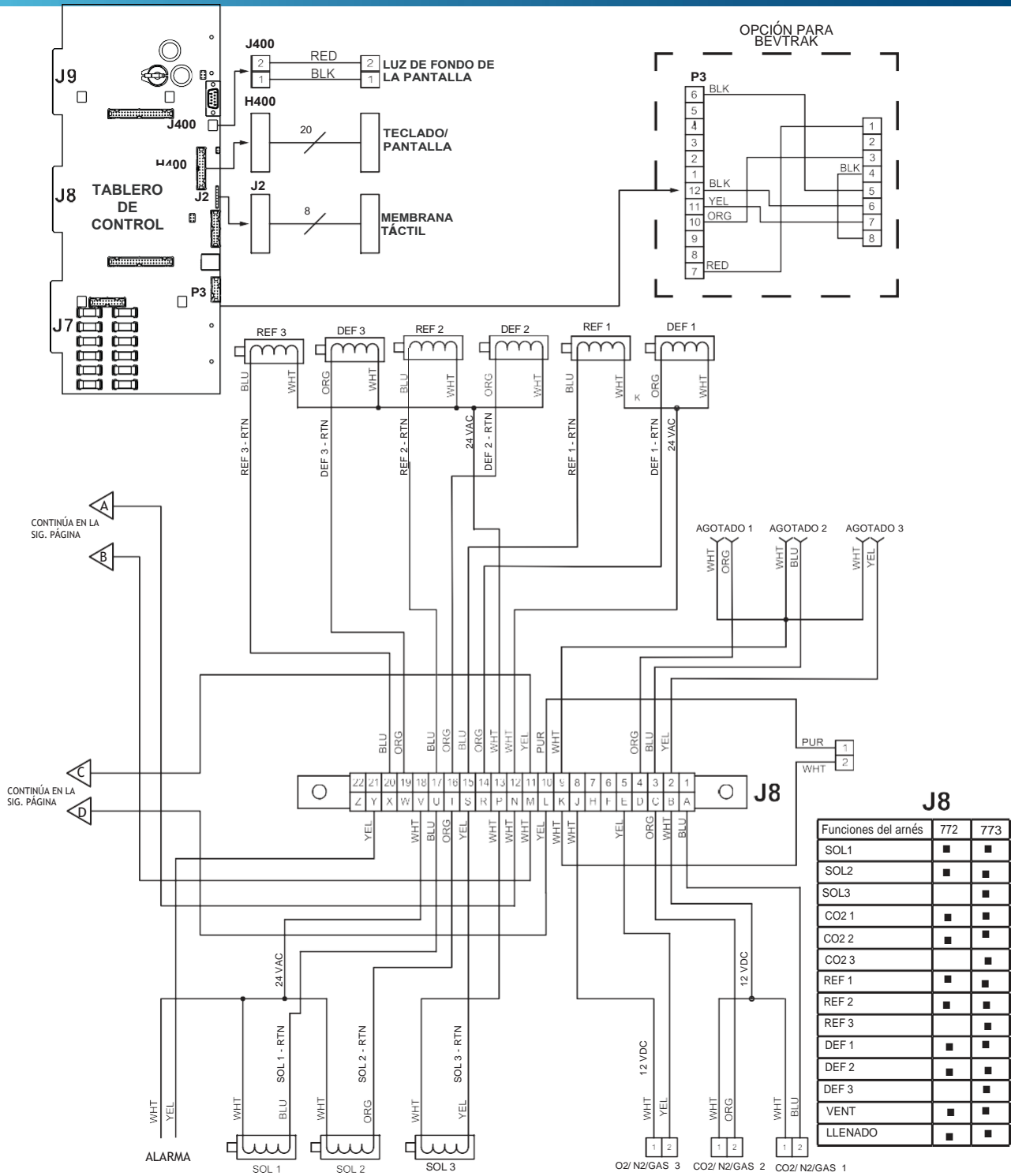
Figura 11.8 Diagrama eléctrico del dispensador estándar 372 2 DE 3
