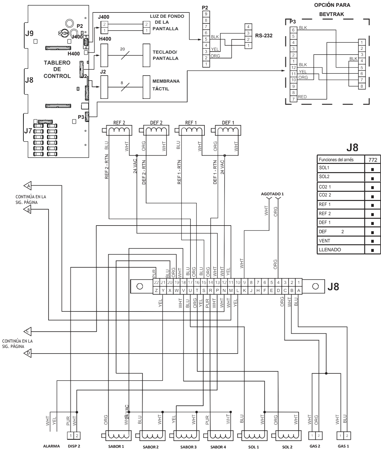
Figura 11.11 Diagrama eléctrico del dispensador de múltiples sabores 372
