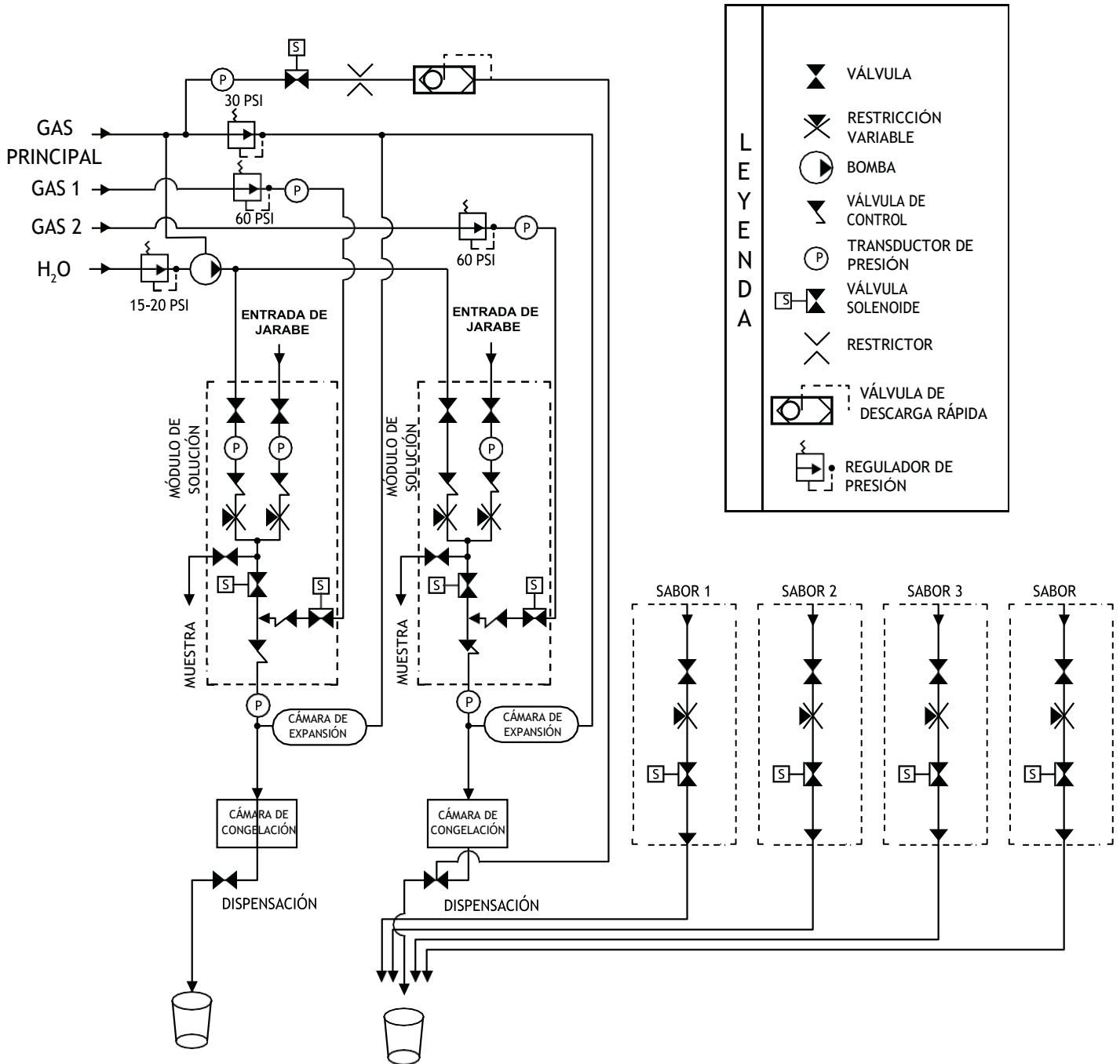
Figura 11.6 Diagrama de flujo del dispensador de múltiples sabores 372
