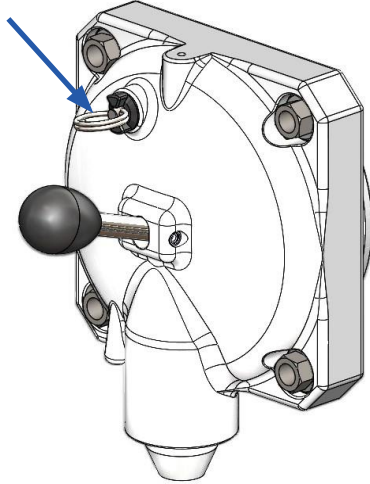
Figura 5.3 Ubicación de la válvula de alivio en varios tipos de placas frontales
