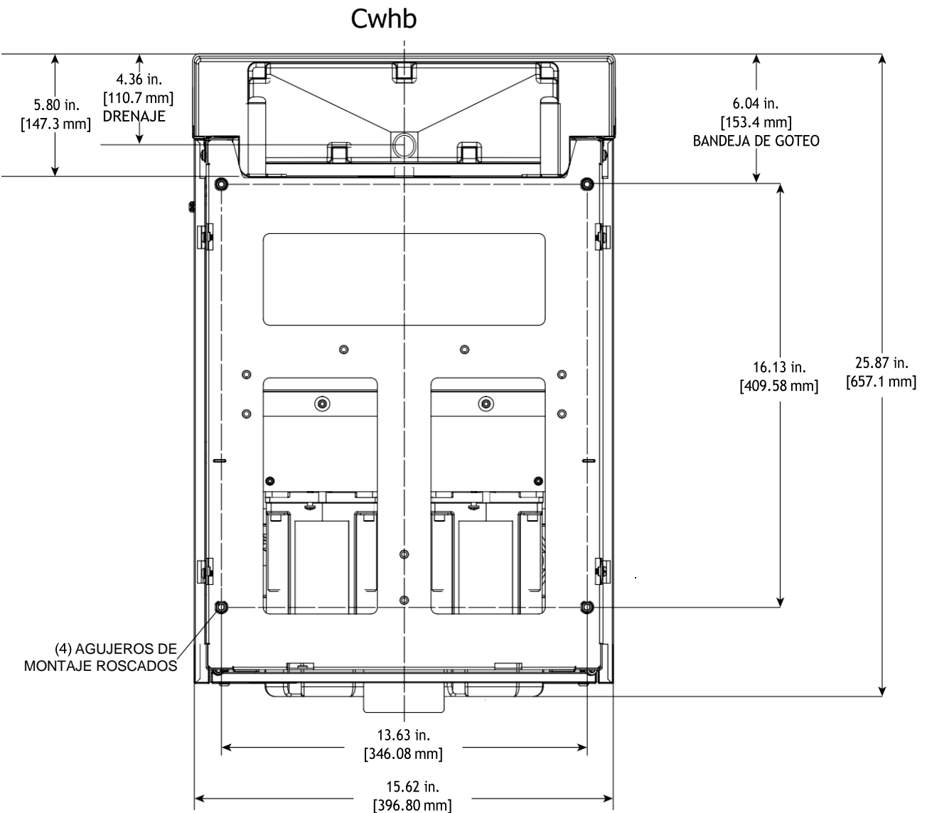
Figura 11.1 Diagrama de montaje del dispensador 372
